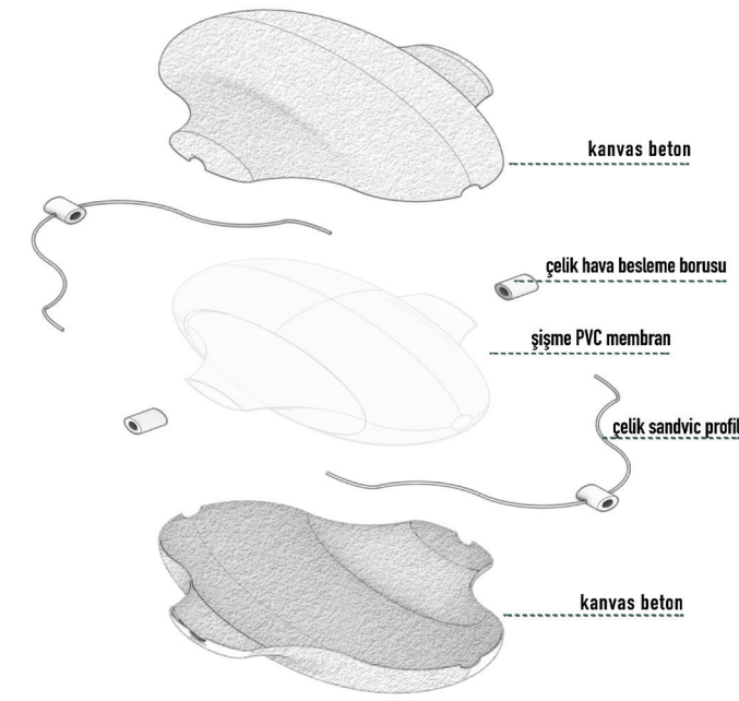
modül detay diyagramı
